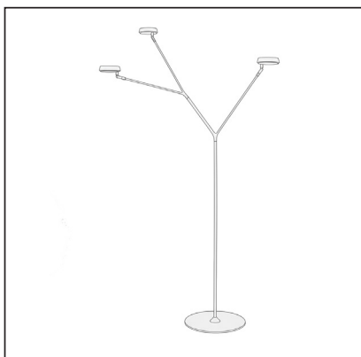
Samenstelling van de tree: metalen plaat, 3 palen met verlengstukken, 3 ledmodules
