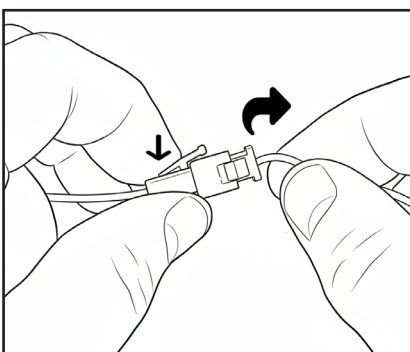
Paso 7: Desconecte la batería presionando la palanca y tirando del cable
