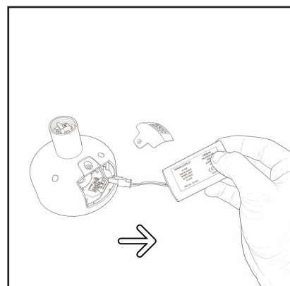
Passaggio 6: Estrarre la batteria
