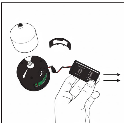
Étape 5 : Sortez la batterie
