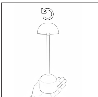
Étape 1 : Tournez la tête de la base ou du poteau dans le sens antihoraire
