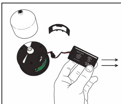
Passaggio 6: Estrarre la batteria
