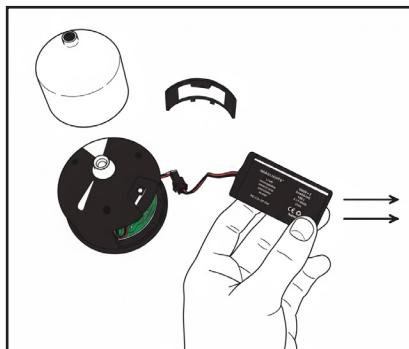
Paso 6: Saque la batería
