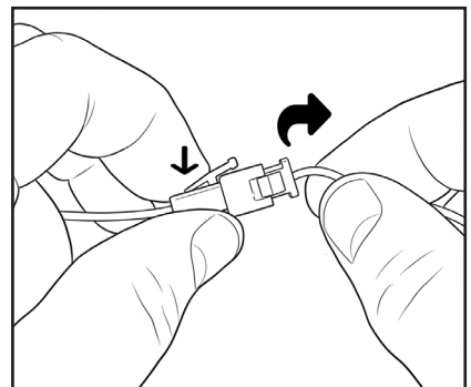
Paso 7: Desconecte la batería presionando la palanca y tirando del cable
