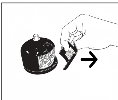
Étape 5 : Retirez la porte en plastique
