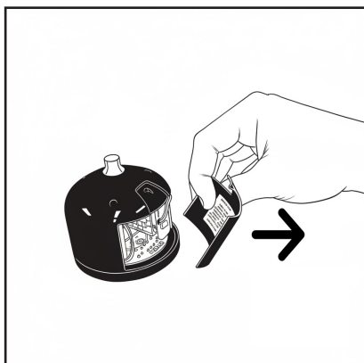
Stap 5: Verwijder het kunststof deurtje
